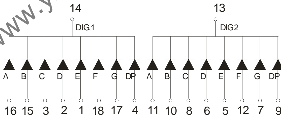
数码管显示及引脚位置图
