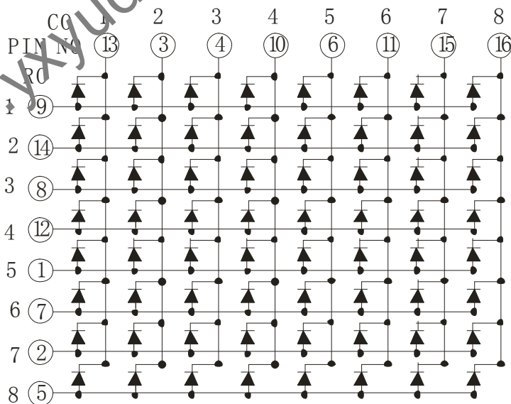
数码管显示及引脚位置图
