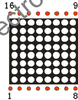
数码管显示及引脚位置图
