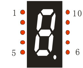
数码管显示及引脚位置图
