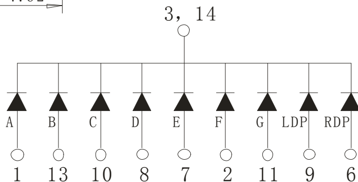
数码管显示及引脚位置图
