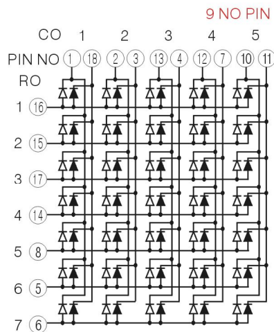
数码管显示及引脚位置图
