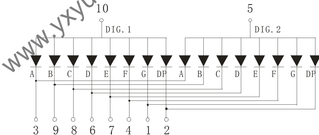
数码管显示及引脚位置图
