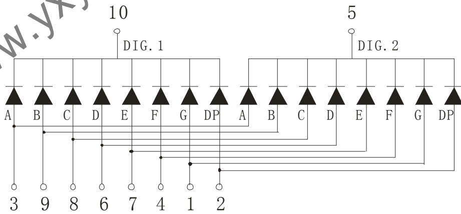
数码管显示及引脚位置图
