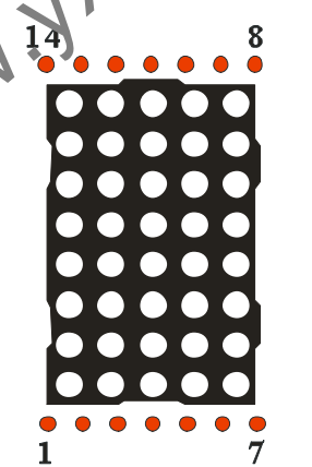
数码管显示及引脚位置图
