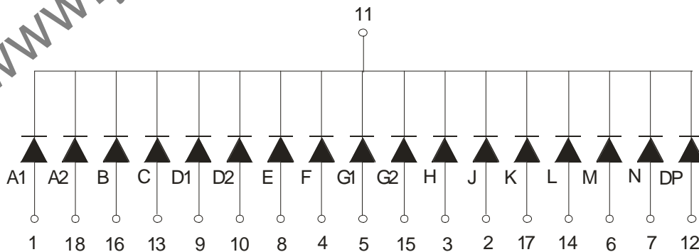
数码管显示及引脚位置图
